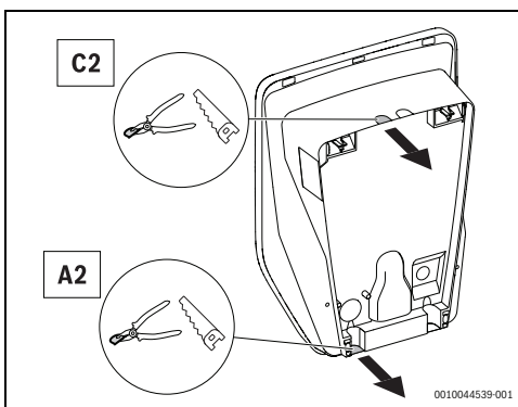
Fig. 154 Capacul racordului electric
