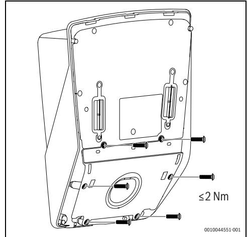
Bild 89 Installation des Parkhalters
