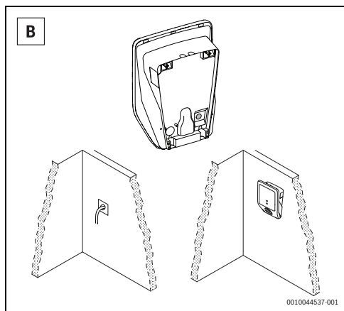
Obr. 175 Prívodné vedenie zo stredu
