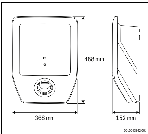
Fig. 148 Dimensiuni produs
