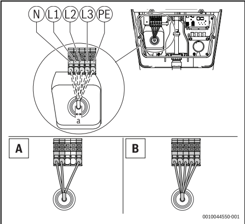
Afb. 37 Elektrische aansluitingen aanvoer A = 1-fasige installatie B = 3-fasige installatie
