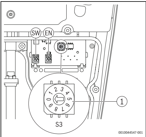
Afb. 38 Keuzetoets max. stroom (S3)
