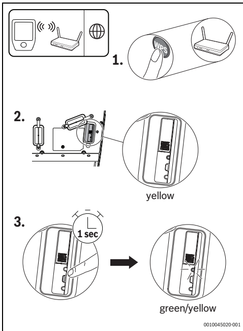
Σχ. 212 Σύνδεση WPS
