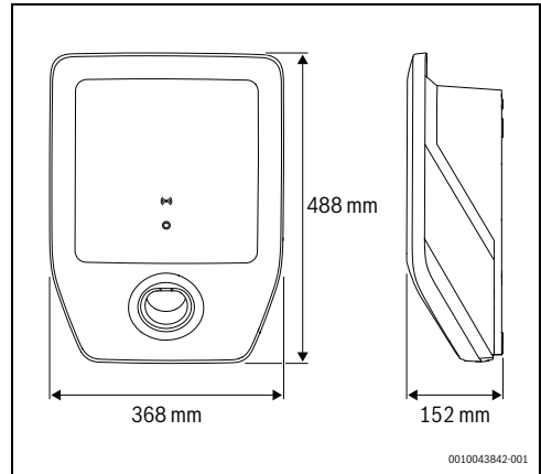
Afb. 28 Productafmetingen
