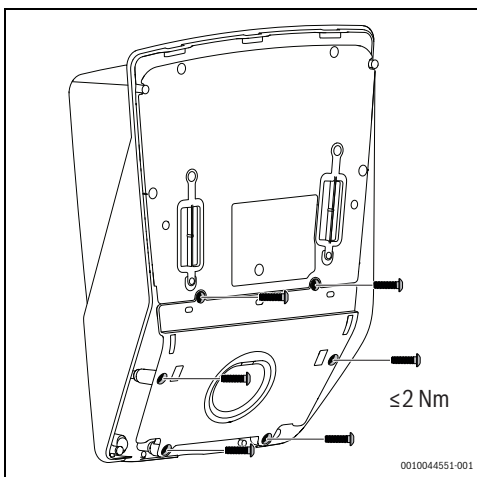
Fig. 161 Instalarea suportului de parcare
