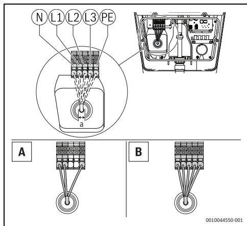
Rys. 133 Podłączenie zasilania elektrycznego
