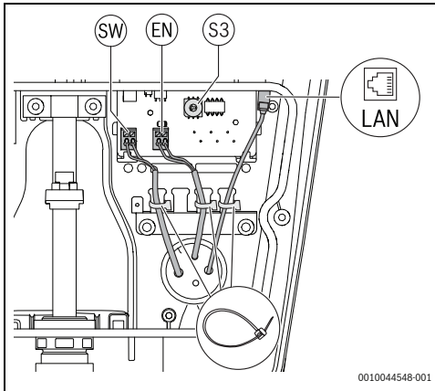
Σχ. 208 Προαιρετικές συνδέσεις εσωτερικής διεπαφής
