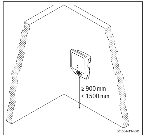
Afb. 29 Minimumafstanden
