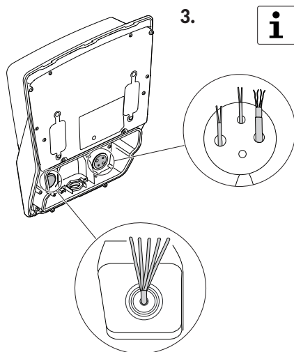
Rys. 132 Montaż na ścianie
