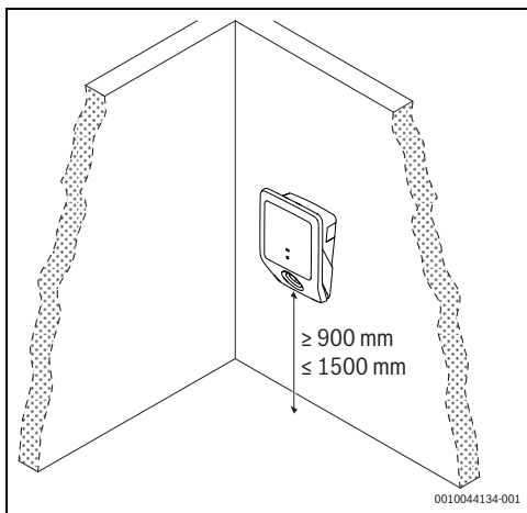
Fig. 149 Distanțe minime
