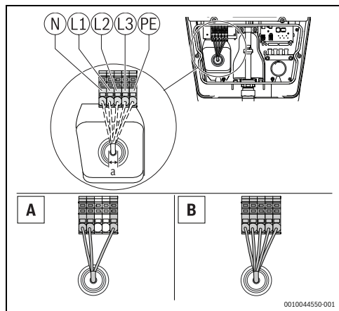
Obr. 181 Prívod elektrických prípojek
