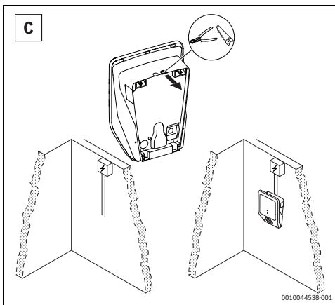
Obr. 8 Napájecí vedení shora
