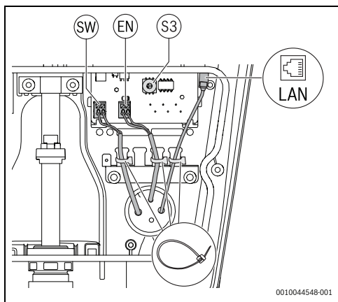
Obr. 16 Volitelná připojení vnitřních rozhraní
