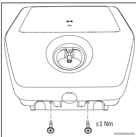
Fig. 162 Instalarea capacului frontal
