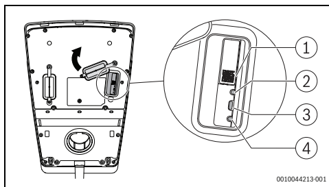
Obr. 171 Prehľad výrobku
