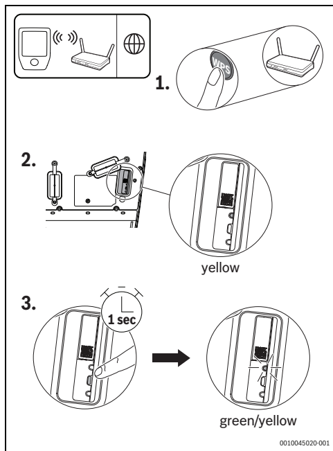
Afb. 44 Verbinding WPS
