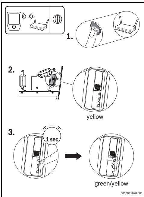
Fig. 68 Connexion WPS
