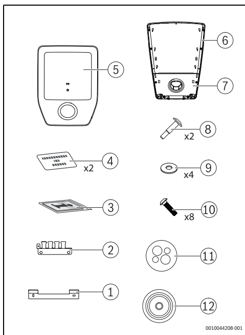
Σχ. 193 Περιεχόμενο συσκευασίας
