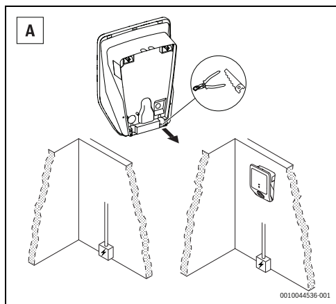
Obr. 174 Prívodné vedenie zospodu
