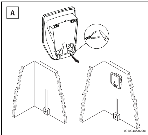
Bild 78 Versorgungsleitung von unten
