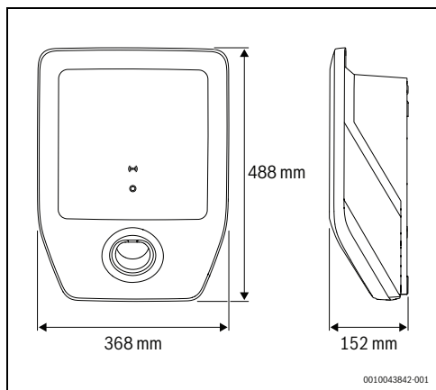
Σχ. 196 Διαστάσεις προϊόντος
