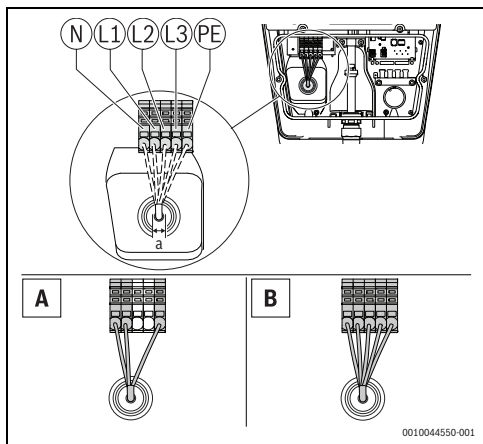
Bild 85 Elektrische Anschlüsse Versorgung A = 1-Phasen-Installation B = 3-Phasen-Installation
