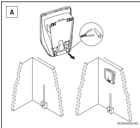
Fig. 102 Linea di alimentazione dal basso
