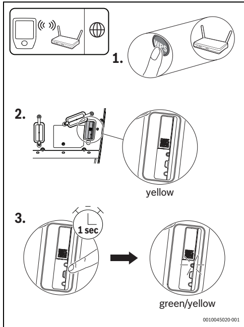
Bild 92 WPS-Verbindung
