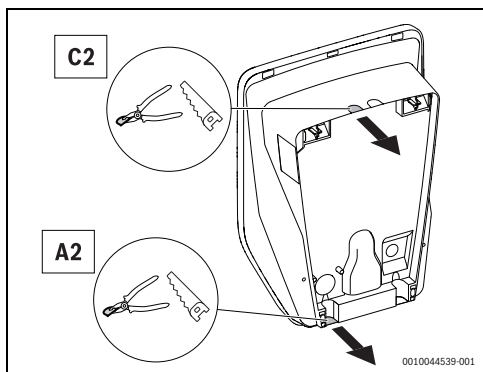
Rys. 130 Zaślepka połączeń elektrycznych
