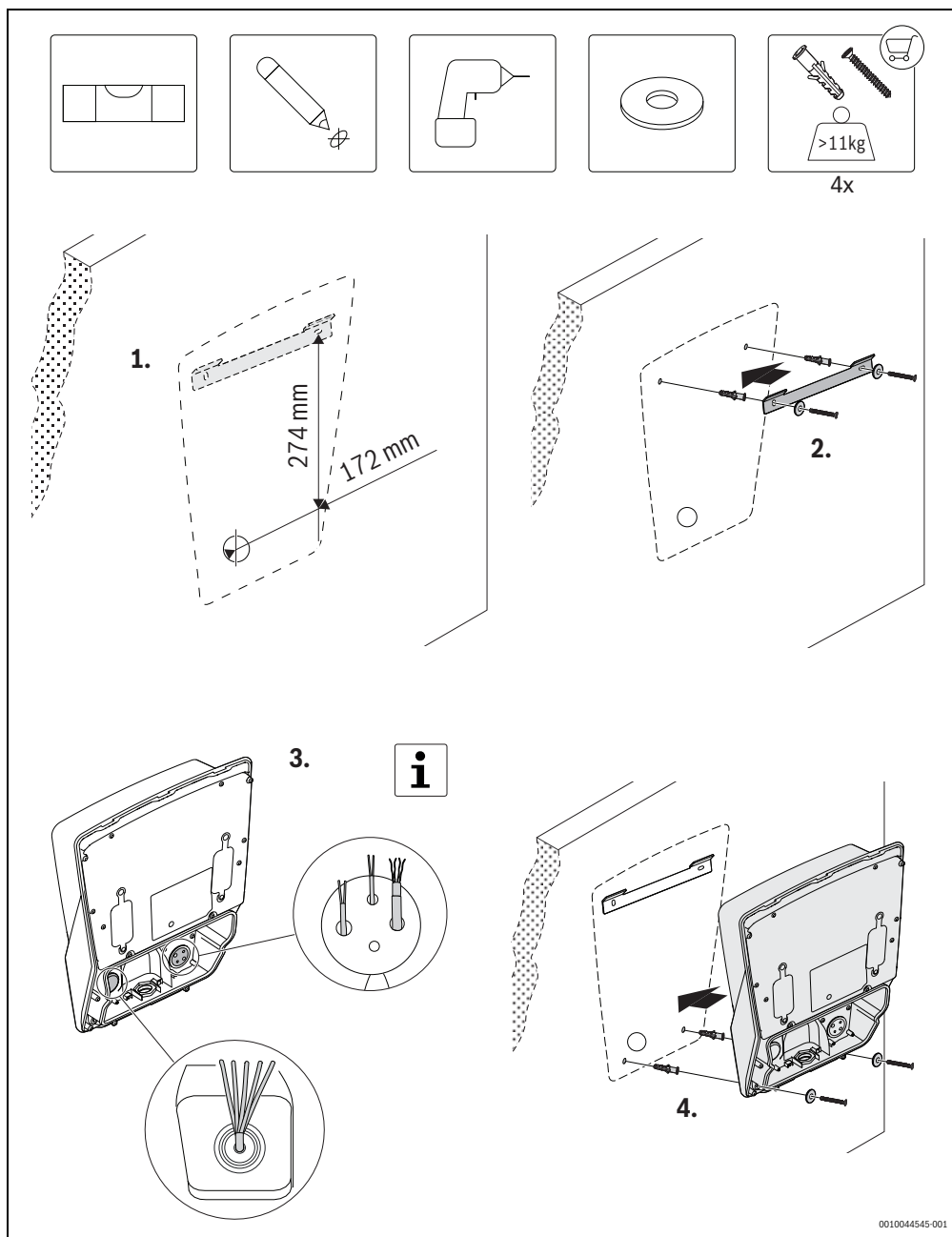
Obr. 180 Montáž na stenu
