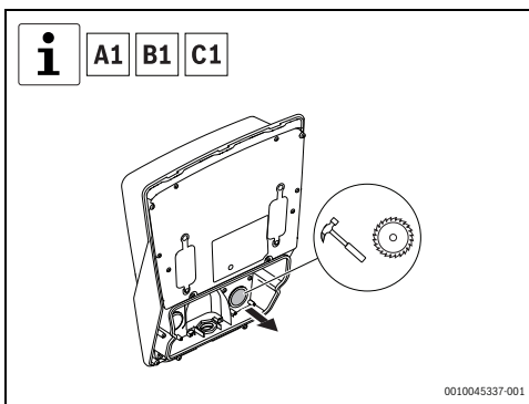
Obr. 9 Odstranění krytu připojení vnitřního rozhraní
