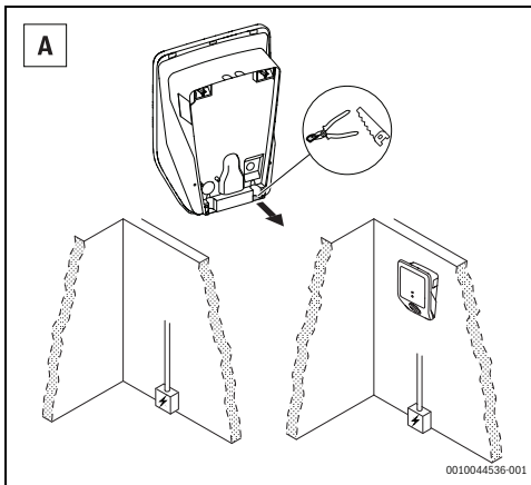
Σχ. 198 Γραμμή παροχή από το κάτω μέρος
