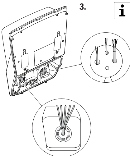
Bild 84 Wandmontage
