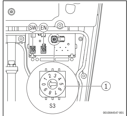
Fig. 158 Buton de selectare al curentului maxim (S3)
