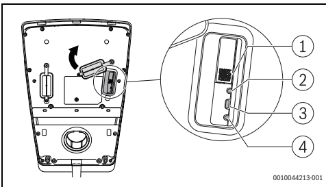
Σχ. 195 Επισκόπηση προϊόντος
