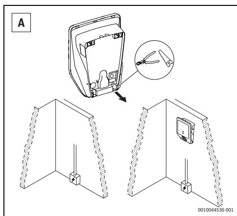
Obr. 6 Napájecí vedení zespodu
