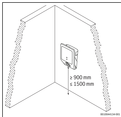
Obr. 5 Minimální vzdálenosti
