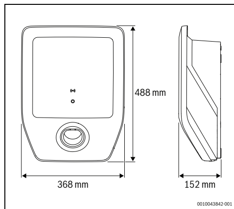
Obr. 4 Rozměry výrobku
