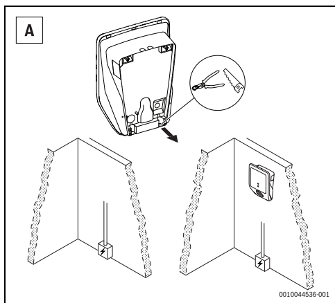
Afb. 30 Voedingsleiding van onderaf
