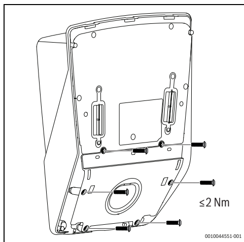
Fig. 65 Installation du support de connecteur
