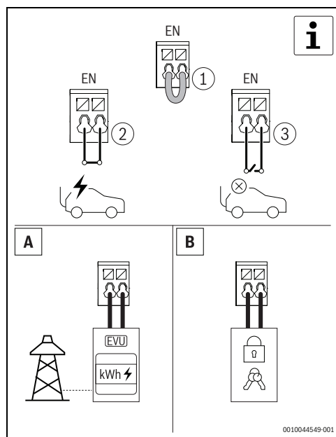
Afb. 47 Optionele digitale input
