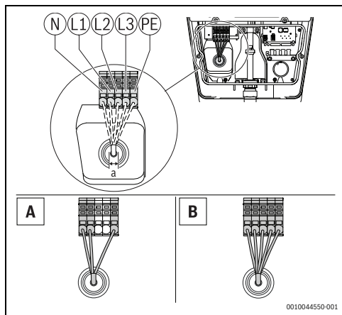
Obr. 13 Napájení elektrického připojení A = 1-fázová instalace B = 3-fázová instalace
