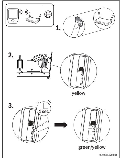
Obr. 188 Pripojenie WPS
