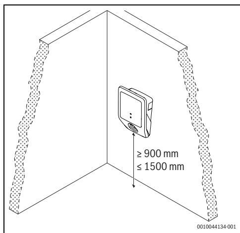
Σχ. 197 Ελάχιστες αποστάσεις
