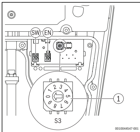
Fig. 62 Bouton de sélection du courant max. (S3)
