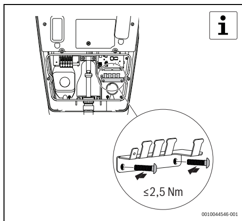
Fig. 159 Instalarea suportului de cabluri
