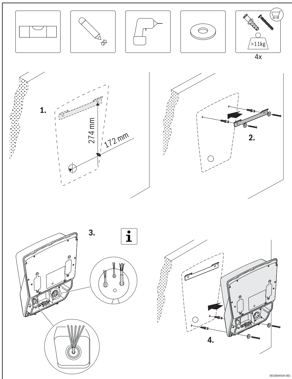
Fig. 156 Montare pe perete
