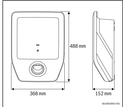
Obr. 172 Rozmery výrobku
