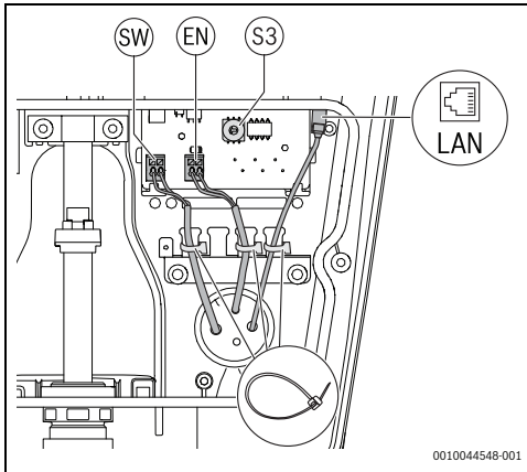
Bild 88 Optionale interne Schnittstellenanschlüsse
