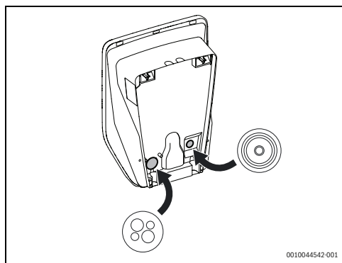
Afb. 35 Installatie van de kabelstopbustule en de kabelstopbus met meerdere gaten (CLIXX)
