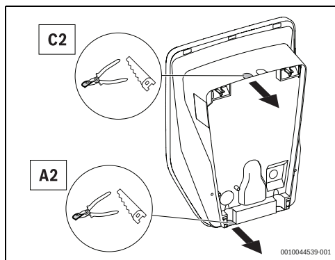
Afb. 34 Dop van elektrische aansluitingen
