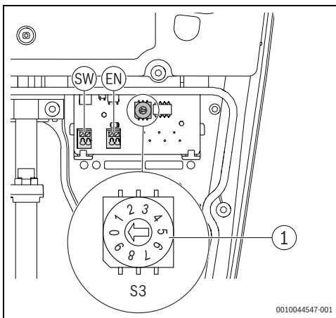
Bild 86 Wahlschalter für max. Strom (S3)
