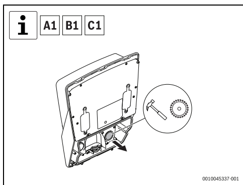
Rys. 129 Wyjmowanie zaślepki połączeń interfejsu wewnętrznego
