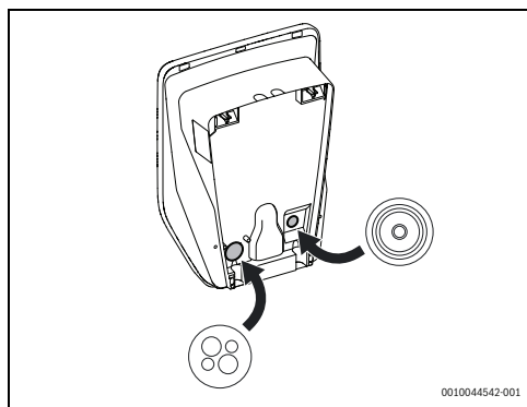
Obr. 179 Inštalácia zátky káblovej prechodky a káblOVEJ prechodky s viacerými otvormi (CLIXX)
