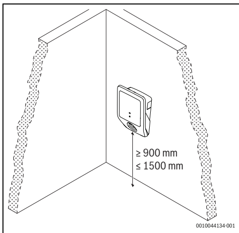
Fig. 53 Dégagements minimaux
