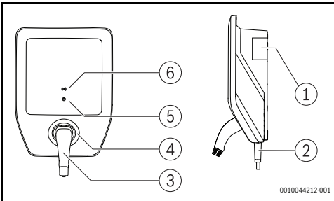
Σχ. 194 Επισκόπηση προϊόντος
