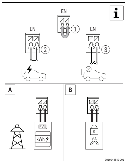
Obr. 23 Volitelný digitální vstup
