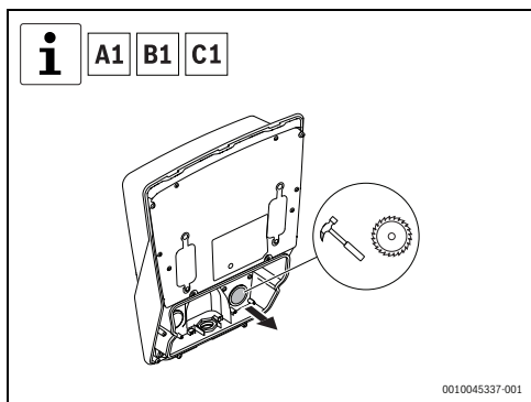
Fig. 153 Îndepărtarea capacului racordului interfeței interne
