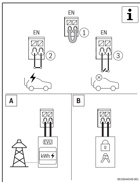
Fig. 167 Intrare digitală opțională
