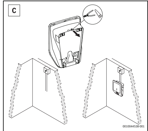
Fig. 104 Linea di alimentazione dall'alto
