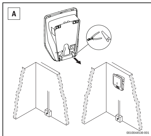
Rys. 126 Przewody zasilania od dołu
