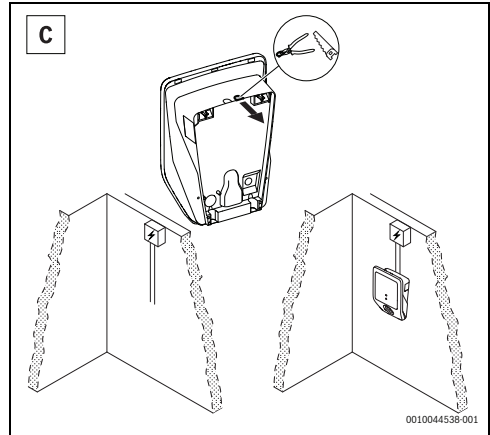
Bild 80 Versorgungsleitung von oben
