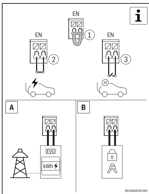
Σχ. 215 Προαιρετική ψηφιακή είσοδος
