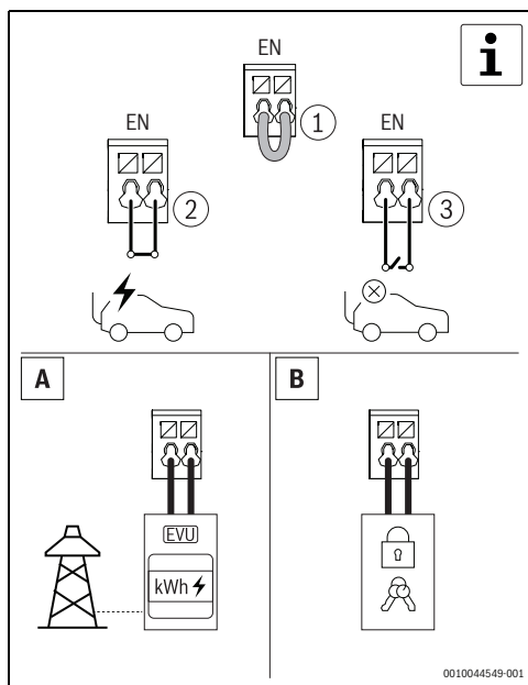
Obr. 191 Voliteľný digitálny vstup
