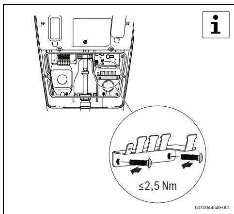
Obr. 15 Instalace držáku kabelu
