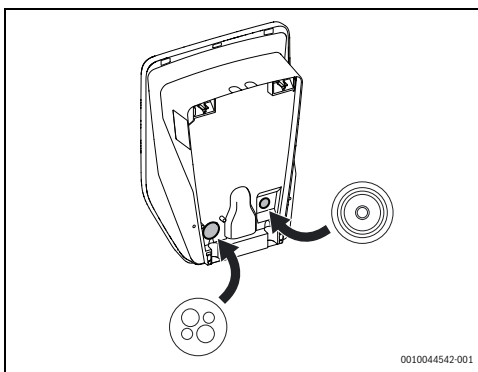
Fig. 155 Instalarea suportului glandei de cablu și glandei de cablu cu multe orificii (CLIXX)
