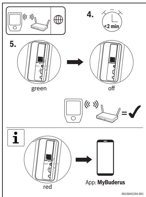
Obr. 21 Připojení WPS
