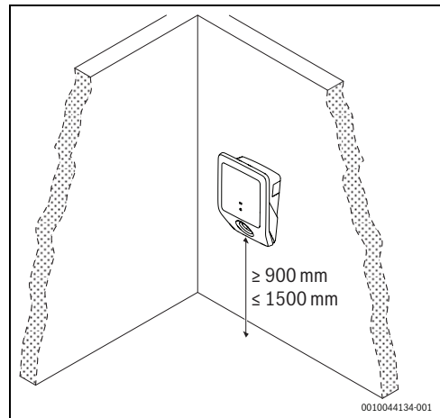
Bild 77 Mindestabstände
