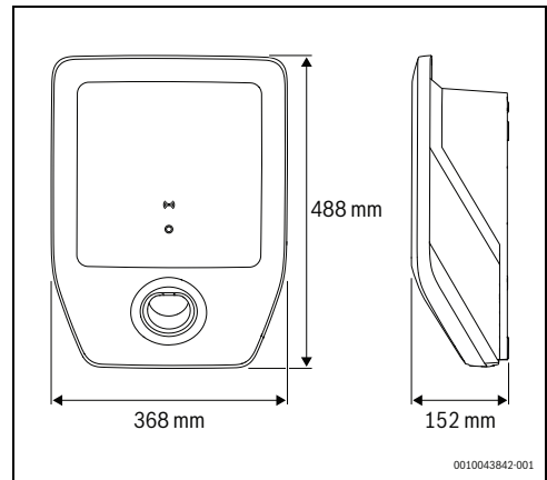
Fig. 52 Dimensions du produit
