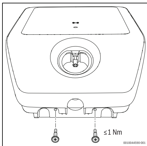
Fig. 66 Montage du cache
