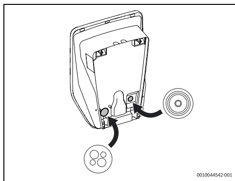
Obr. 11 Instalace těsnění kabelové průchodky a kabelové průchodky s více otvory (CLIXX)
