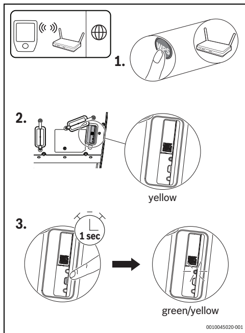
Fig. 164 Racord WPS
