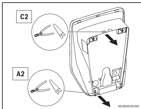
Fig. 58 Capuchon des raccordements électriques
