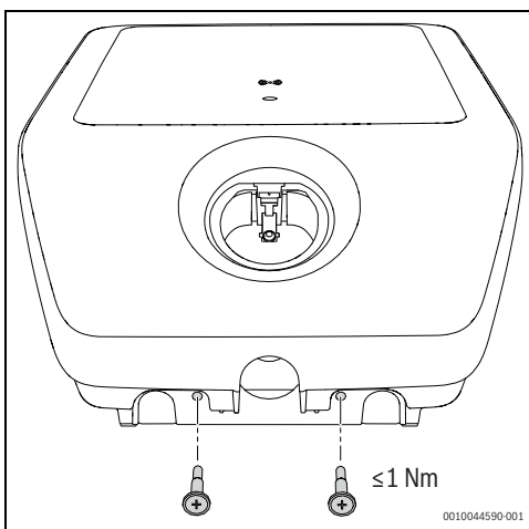
Obr. 18 Instalace čelního krytu
