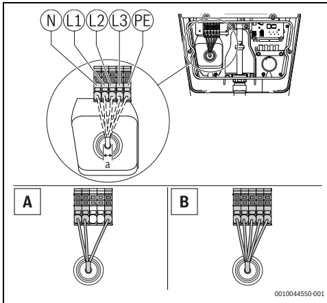
Fig. 157 Alimentarea conexiunilor electrice A = instalație monofazată B = instalație trifazată
