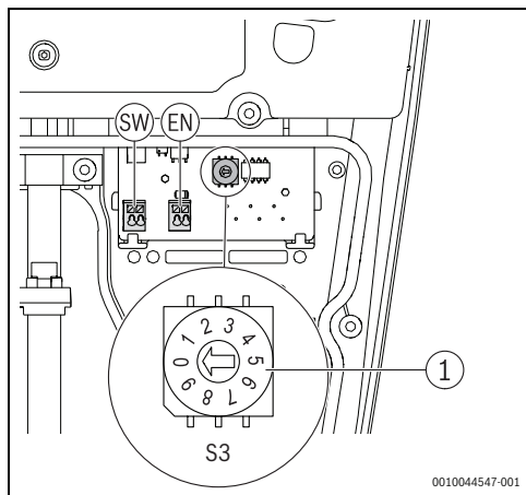
Obr. 182 Volič max. prúdu (S3)
