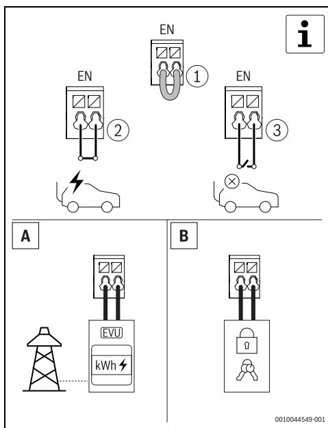
Fig. 71 Entrée numérique en option
