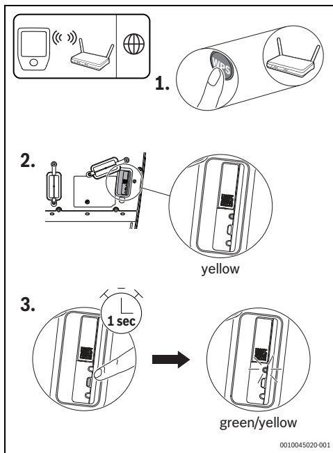
Rys. 140 Połączenie WPS
