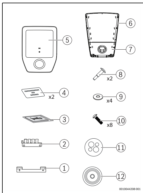
Obr. 169 Rozsah dodávky
