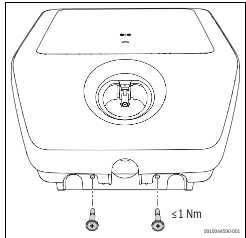
Σχ. 210 Εγκατάσταση μπροστινού καλύμματος
