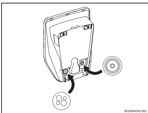
Rys. 131 Montaż pierścienia przelotowego dławika kablowego i wielootworowego dławika kablowego (CLIXX)
