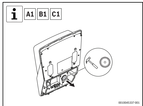
Bild 81 Entfernen der Kappe der internen Schnittstellenanschlüsse
