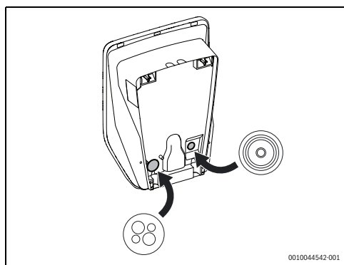
Fig. 59 Installation de la gaine du presse-étoupe de câbles et du presse-étoupe de câbles à trous (CLIXX)
