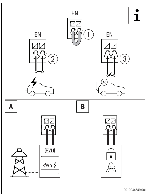
Rys. 143 Opcjonalne wejście cyfrowe
