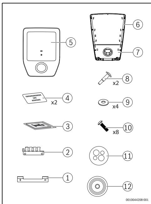
Afb. 25 Leveringsomvang
