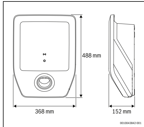
Bild 76 Produktabmessungen
