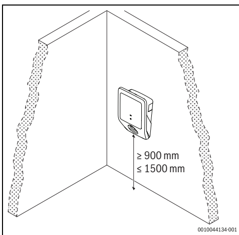
Rys. 125 Minimalne odległości
