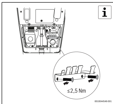
Fig. 63 Montage du porte-câble
