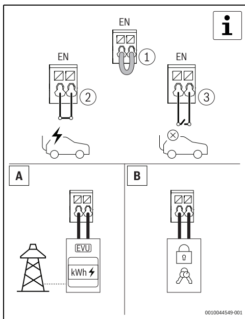
Fig. 119 Ingresso digitale opzionale
