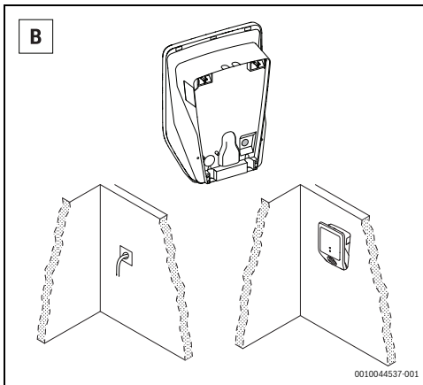
Bild 79 Versorgungsleitung von der Mitte
