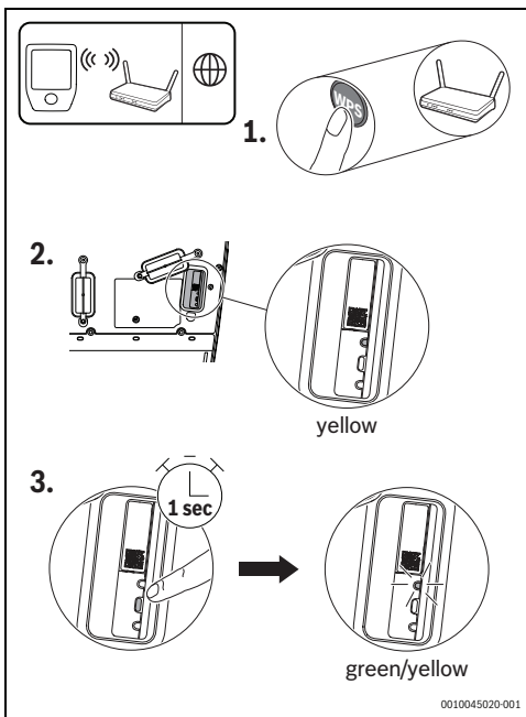
Fig. 116 Collegamento WPS
