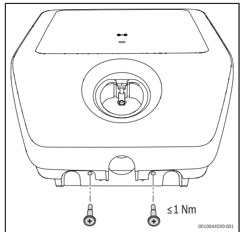
Bild 90 Installation der Abdeckung
