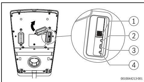
Obr. 3 Přehled výrobku
