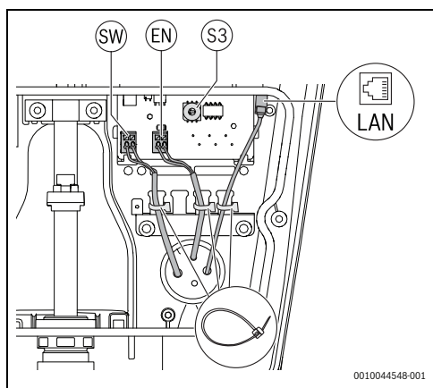
Afb. 40 Optionele interne interfaceaansluitingen
