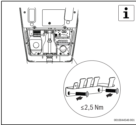
Bild 87 Installation des Kabelhalters
