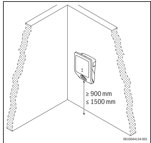
Obr. 173 Minimálne odstupy
