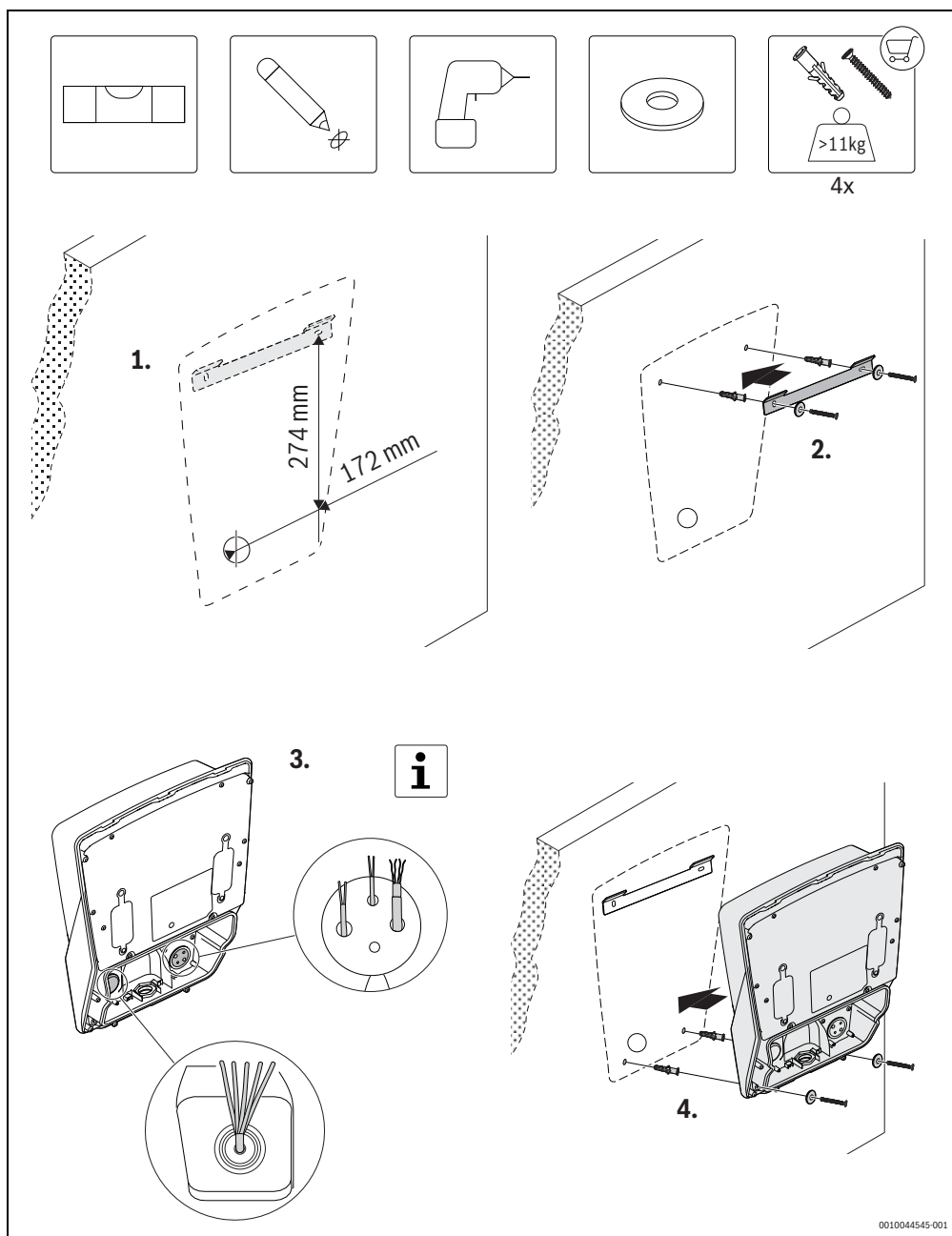
Fig. 108 Montaggio a parete
