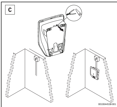
Afb. 32 Voedingsleiding van bovenaf
