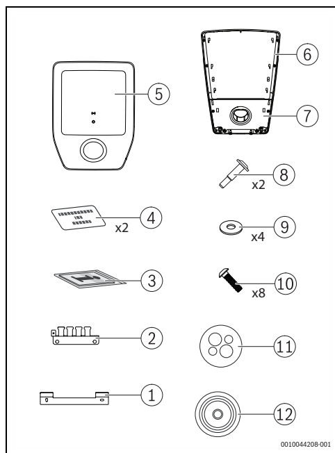
Rys. 121 Zakres elementów
