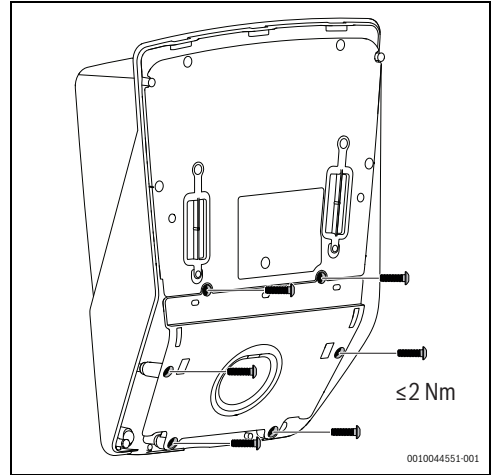
Σχ. 209 Εγκατάσταση βάσης τοποθέτησης
