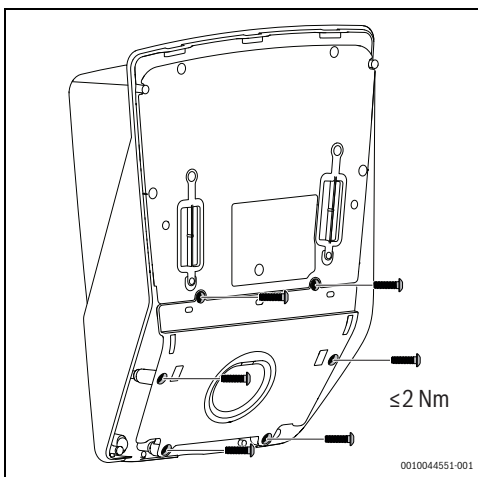
Obr. 17 Instalace parkovacího držáku
