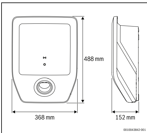
Rys. 124 Wymiary produktu
