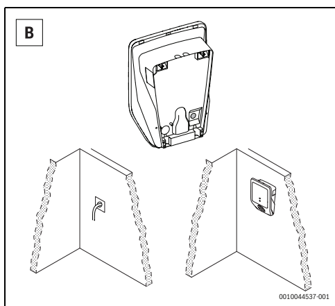
Afb. 31 Voedingsleiding vanaf het midden
