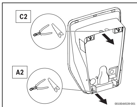
Obr. 10 Kryt elektrických připojení
