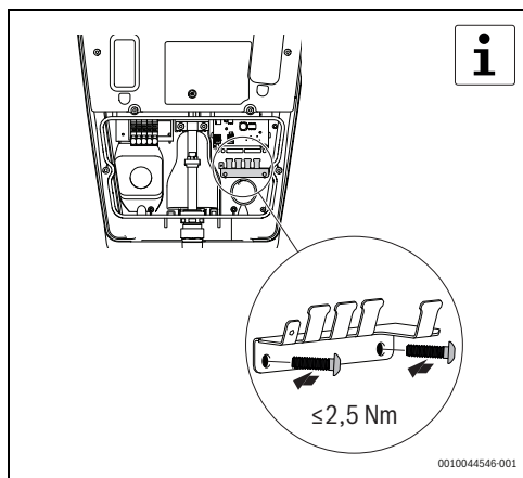
Rys. 135 Montaż uchwyty kabla
