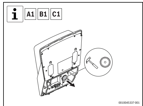
Σχ. 201 Αφαίρεση του καπακιού των συνδέσεων εσωτερικής διεπαφής
